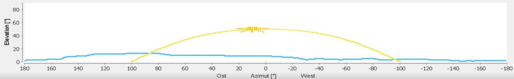
Sonnenbahn und Horizont
